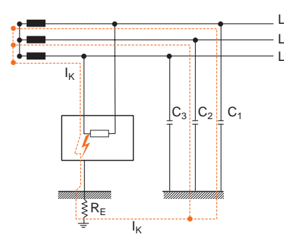
Fig.8: guasto a terra in un sistema IT
