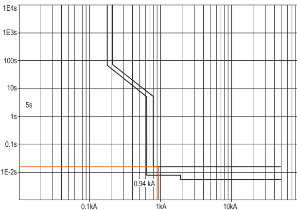
Curva di intervento T2S160 PR221DS-LS/ In160
