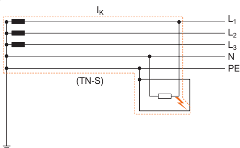
Fig.6: guasto a terra in un sistema TN
