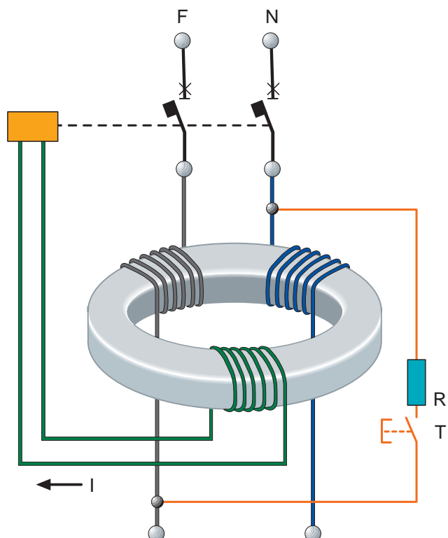
Fig. 6: principio di funzionamento del relè differenziale
