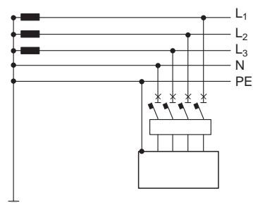
Fig. 5: principio di funzionamento della funzione G
