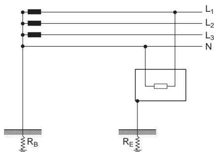
Fig.1: sistema TT
