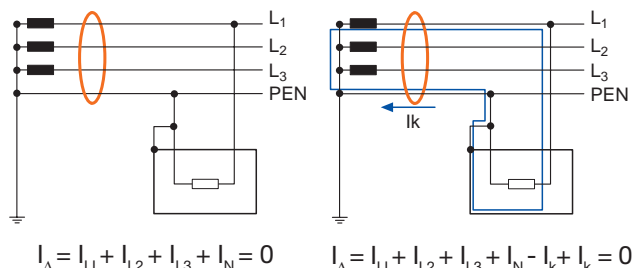
Fig.14: differenziale nel sistema TN-C
