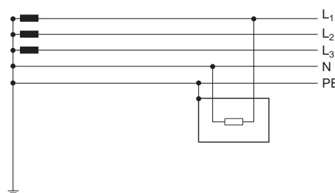
Fig.3: sistema TN-S
