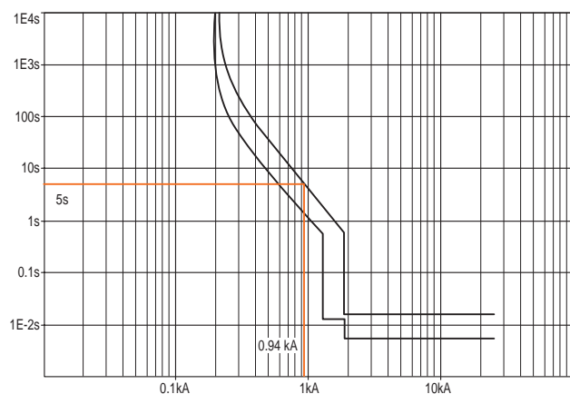
Curva di intervento Tmax T1C160 In160
