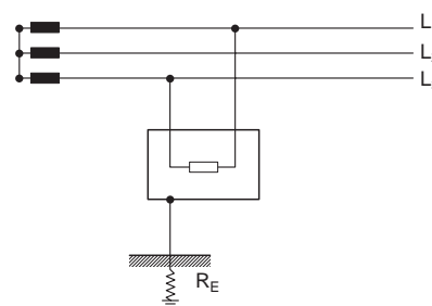
Fig.7: sistema IT
