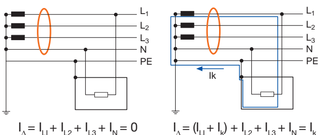
Fig.13: differenziale nel sistema TN-S
